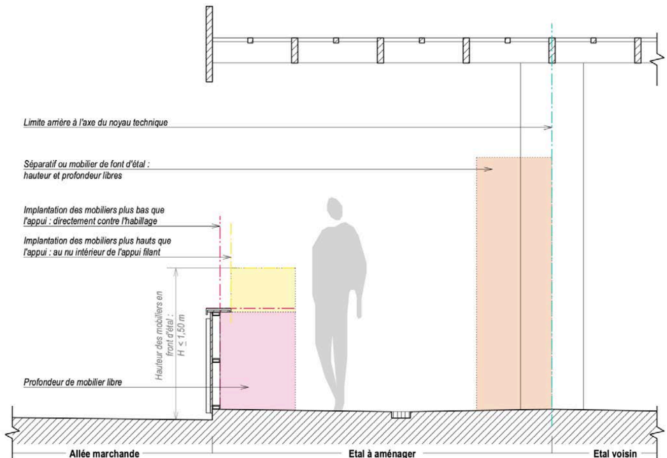
Figure 7 - Coupe de principe des volumes de mobilier à l'intérieur de l'étal fixe
