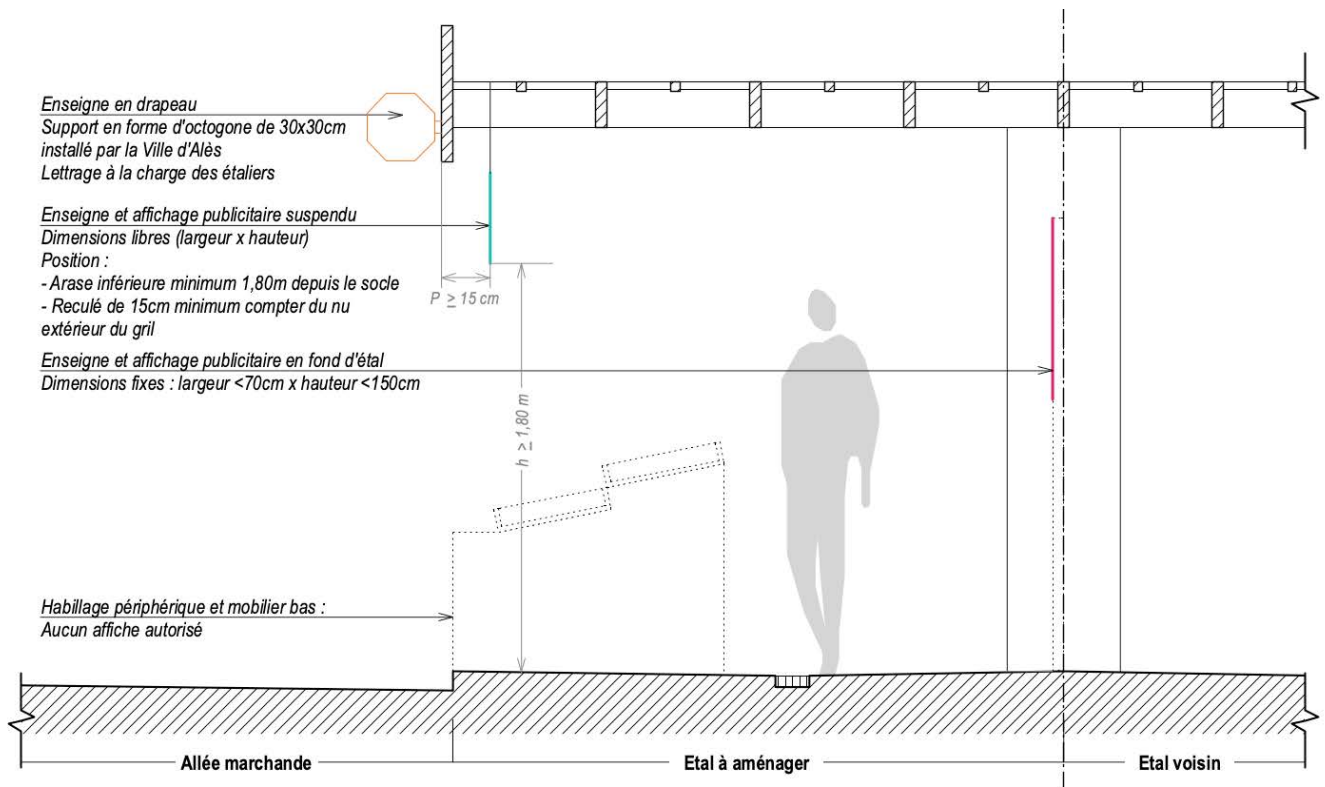
Figure 19 - Coupe schématique de la localisation et dimension de la signalétique autorisée
