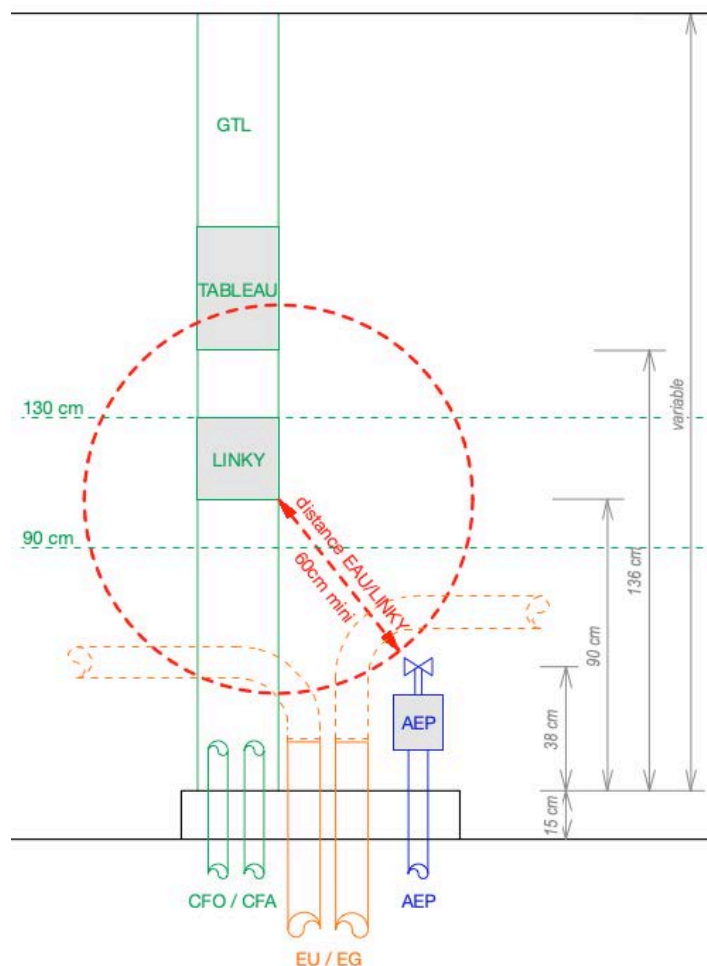
Figure 33 - Coupe schématique illustrant la localisation des attentes au sein d'une borne technique
