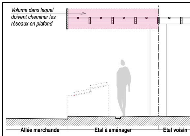
Figure 15 - Coupe schématique illustrant le volume délimité par le grill
