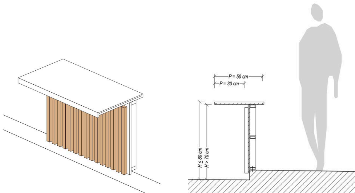
Figure 10 – Vue 3D et coupe sur le plan PMR
