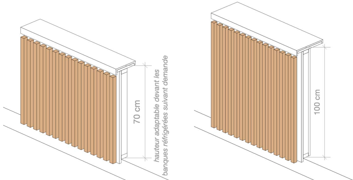
Figure 8 – Visuel de principe de l'habillage périphérique (habillage standard à gauche, plan bar à droite)
