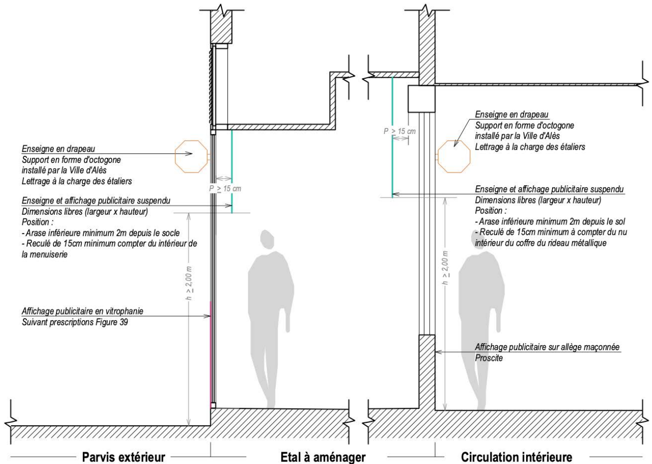
Figure 34 - Coupe schématique de la localisation de la signalétique en façades extérieure (gauche) et intérieure (droite)
