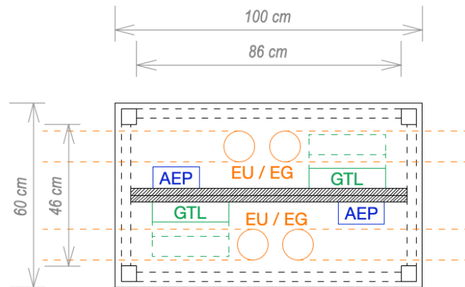
Figure 17 - Plan schématique illustrant la localisation des attentes au sein d'une borne technique
