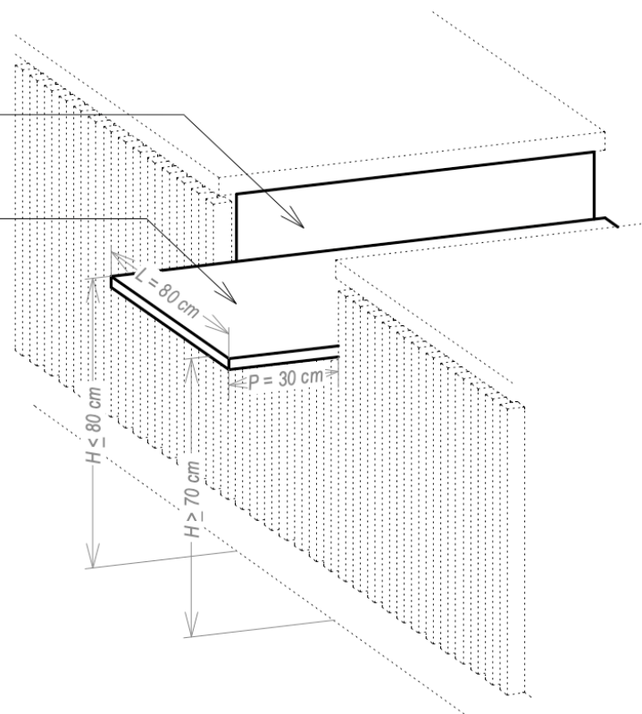
Figure 25 - Croquis du principe à respecter pour le plan accessible PMR à l'intérieur de l'étal
