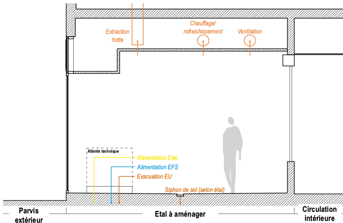
Figure 31 - Schéma illustrant la localisation des réseaux en attente à disposition
