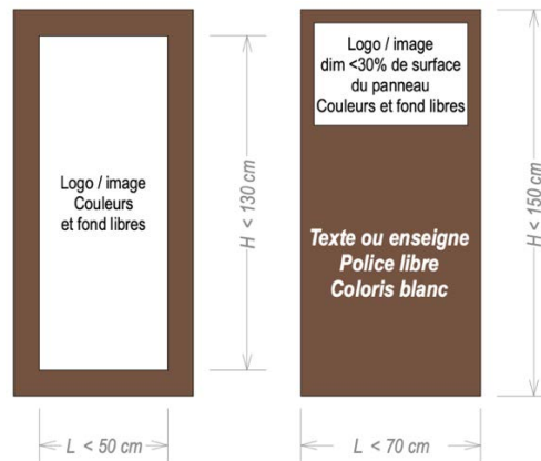
Figure 37 – Schéma des panneaux autorisés en fond d'étal
