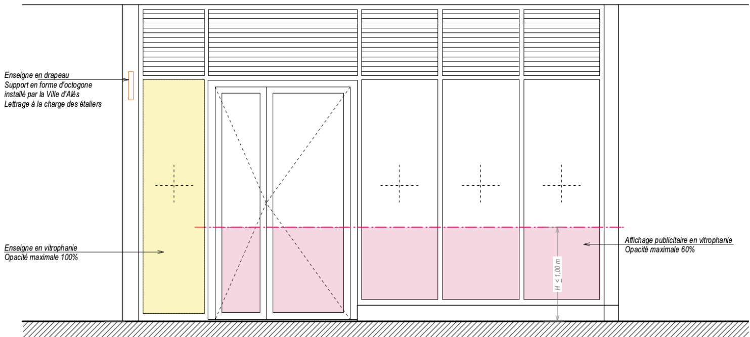
Figure 38 - Élévation schématique de la localisation autorisée de la signalétique en façade sur rue
