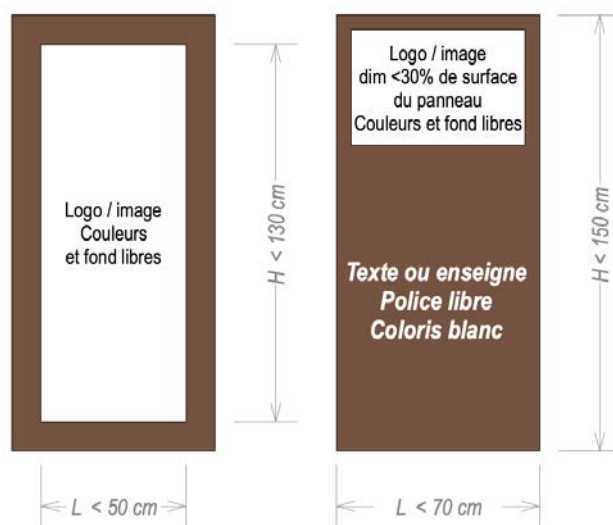
Figure 22 – Schéma des panneaux autorisés en fond d’étal
