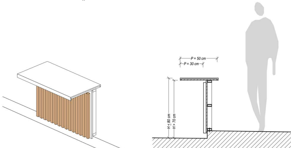
Figure 29 - Croquis du principe à respecter pour la banque PMR accessible depuis l'intérieur des Halles
