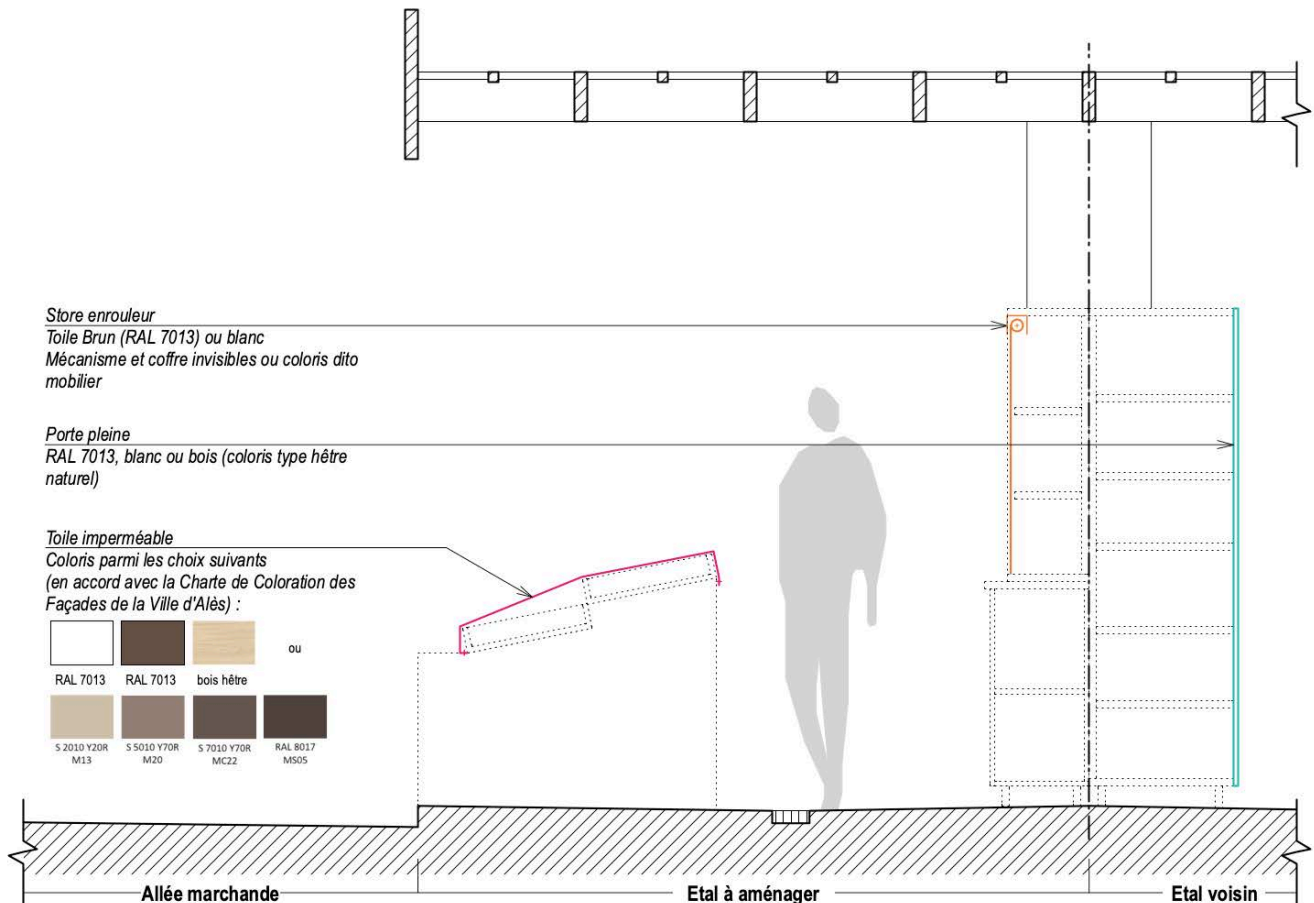
Figure 12 - Coupe de principe des différents systèmes de fermeture en fonction du type de mobilier
