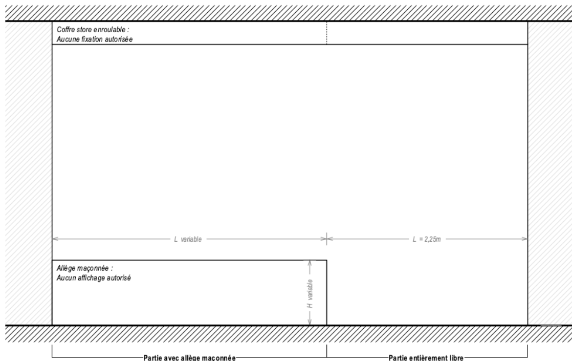
Figure 26 - Croquis d'une façade type d'un étal traversant sur l'intérieur des Halles
