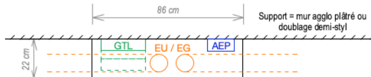
Figure 32 - Plan schématique illustrant la localisation des attentes au sein d'une borne technique
