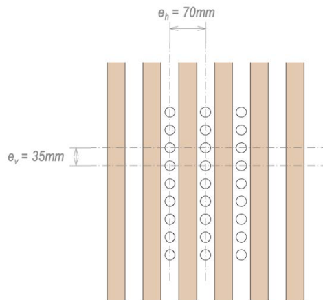
Figure 13 – Schéma des percements autorisés sur l'habillage périphérique
