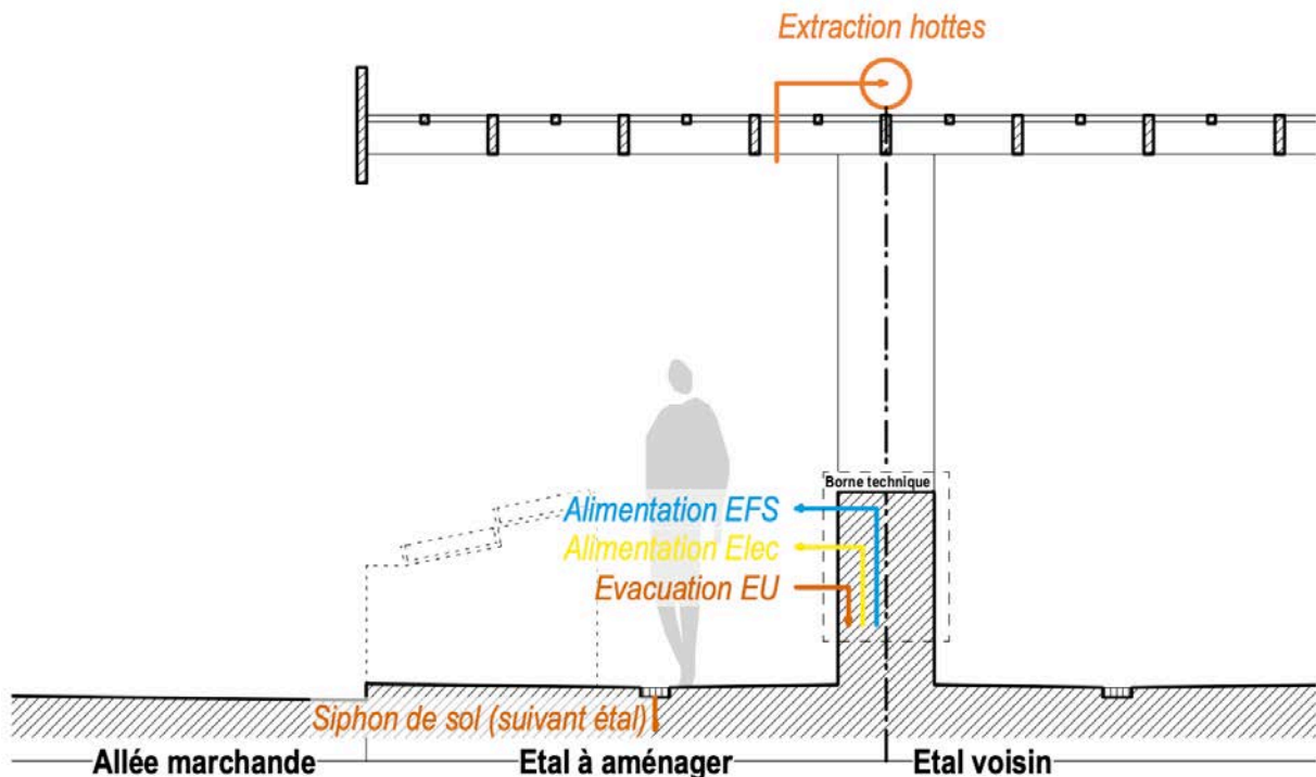
Figure 16 - Schéma illustrant la localisation des différentes attentes à disposition
