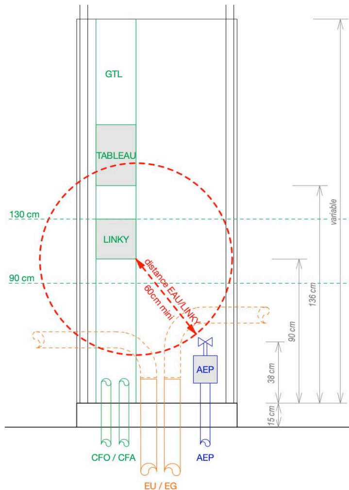
Figure 18 - Coupe schématique illustrant la localisation des attentes au sein d'une borne technique
