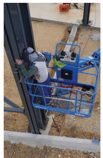
1 Cinq ouvriers spécialisés ont assuré un travail d'équilibriste, parfois jusqu'à 14 mètres au-dessus du sol, pour boulonner les poutres.
